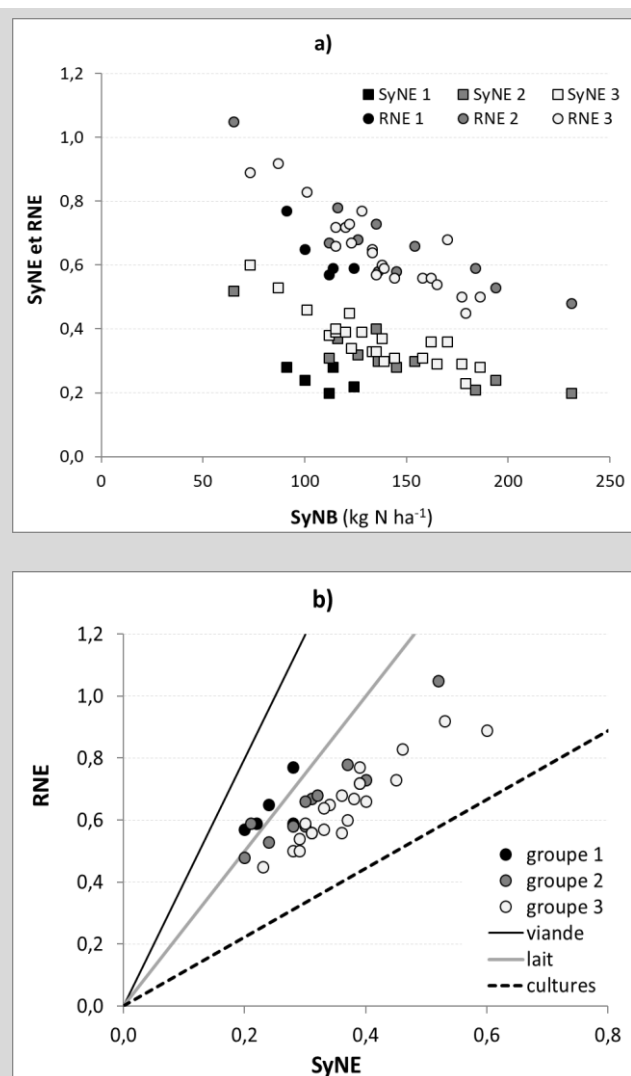
FIGURE 5 : Relation entre les indicateurs d'efficacité SyNE et RNE, et les excédents d'azote SyNB (a) ; relation entre les deux nouveaux indicateurs d'efficacité d'utilisation de l'azote, RNE et SyNE (b).
